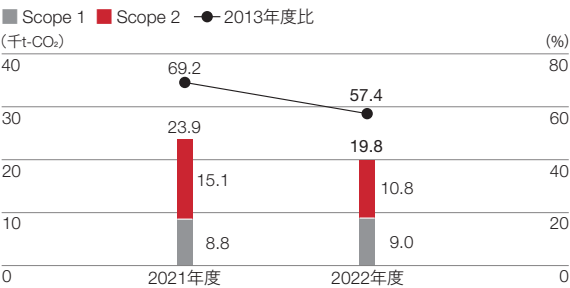
温室効果ガスの排出量の推移
