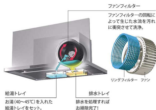
ファンフィルターの構造
