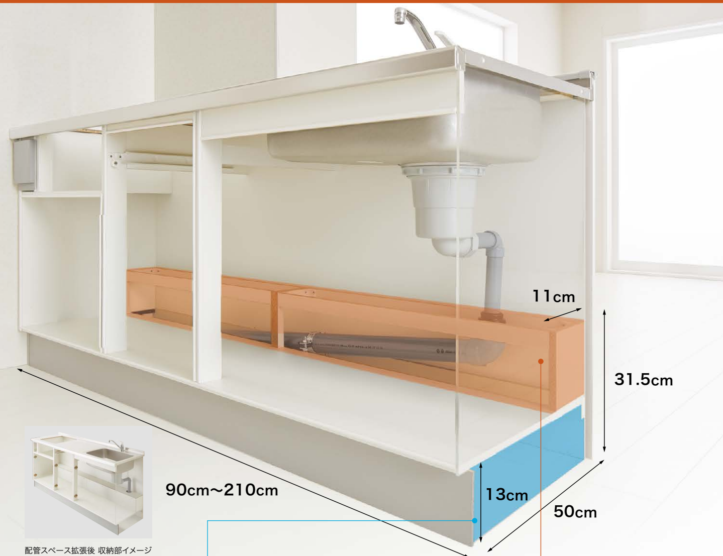
配管スペース拡張後 収納部イメージ
