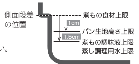
キャセロール断面図
